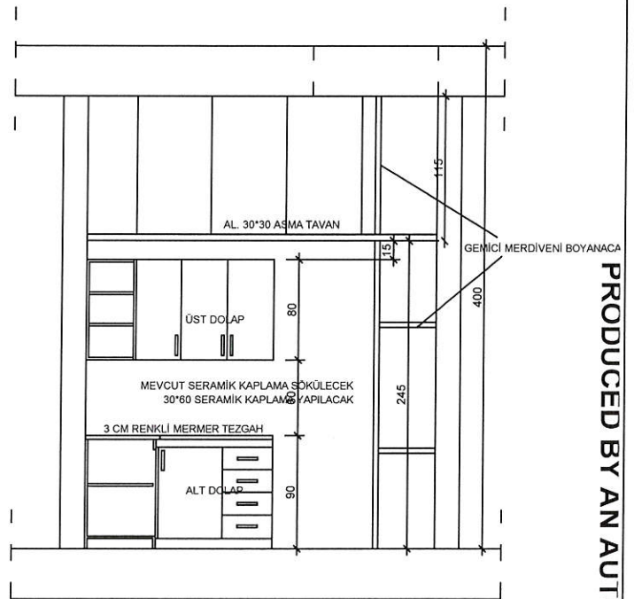
BB KESİTİ
